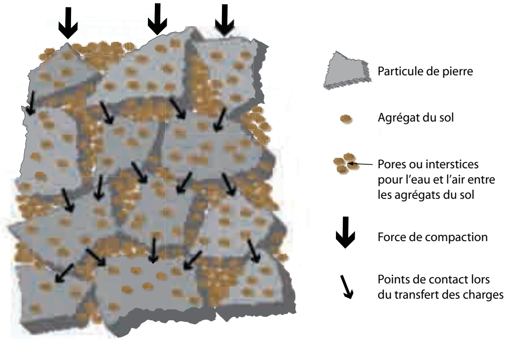
Figure 7. Diagramme conceptuel de sol structural montrant le principe de la compaction pierre-sur-pierre et les espaces interstitiels remplis de sol.
