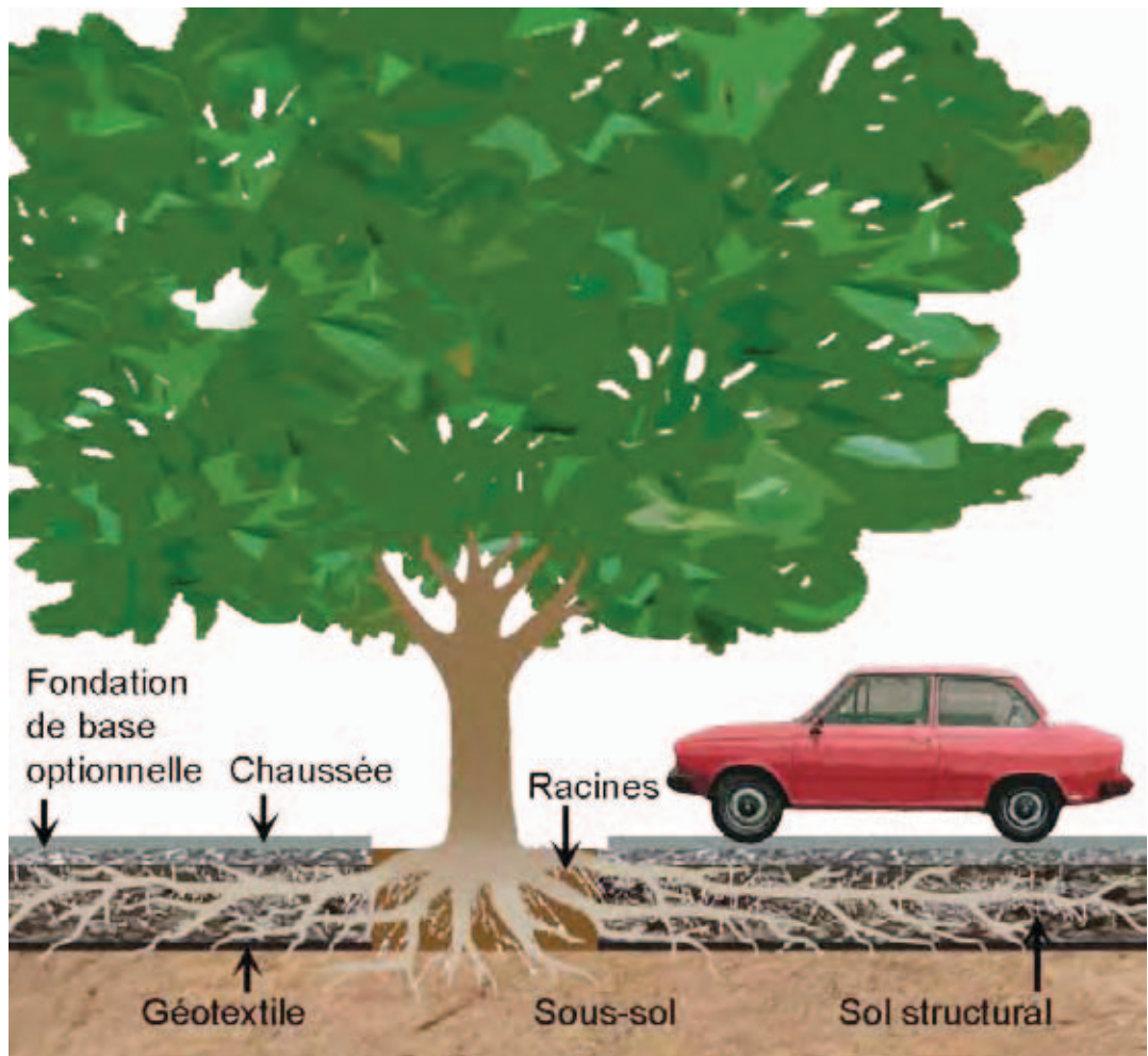
Figure 2. Ce système sert à la fois de stationnement et d'installation de gestion des eaux pluviales. En plus de cette double utilisation de l'espace, les sols structuraux offrent un volume de sol grandement supérieur pour la croissance des racines des arbres que les stationnements construits selon les méthodes traditionnelles.
