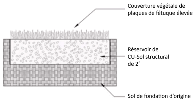
Figure 15. Coupe type d'un gazon renforcé de pelouse en plaque sur sol structural. N.B. La profondeur de 24'' du réservoir se base sur les données pluviométriques locales et est susceptible de varier selon les régions en fonction des données pluviométriques locales et/ou des quantités d'eaux de ruissellement anticipées.
